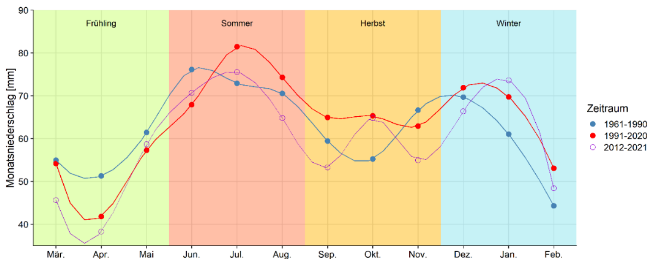
Abbildung 16: Vergleich des mittleren monatlichen Niederschlags in Niedersachsen für die Zeiträume 1961-1990, 1991-2020 und 2012-2021 (aktueller 10-jähriger Zeitraum). Datengrundlage: HYRAS-DE-PRE.
