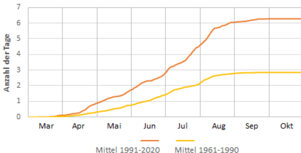
Abbildung 60: Summierte Anzahl Tage mit Waldbrandgefahrenindex WBI \geq 4 ab 01.03. bis 31.10 eines Jahres im Mittel für Niedersachsen 1961-1990 (Gelb) sowie 1991-2020 (Orange). Datengrundlage: DWD.
